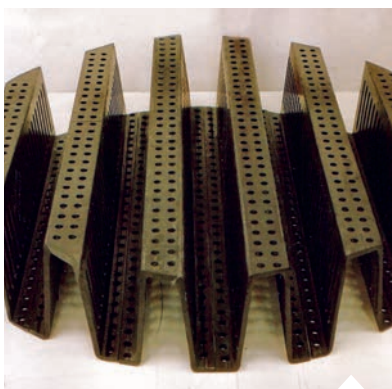
GVK trapeziumrooster voor luchtverdeling
