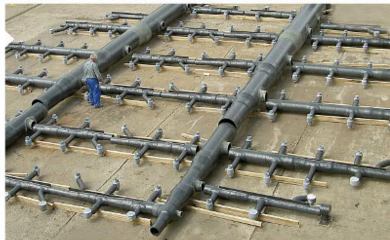
Sprühebene Absorber
